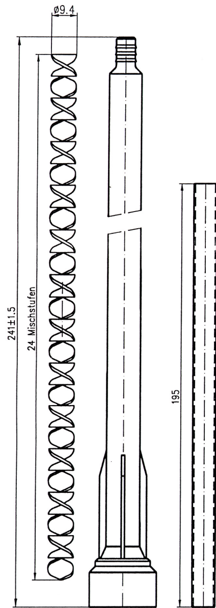
ZM 24 A Verlängerung extension
