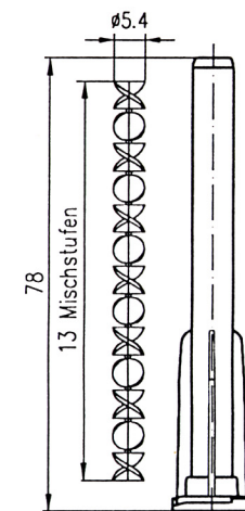
Mischer SM 5,4x13
